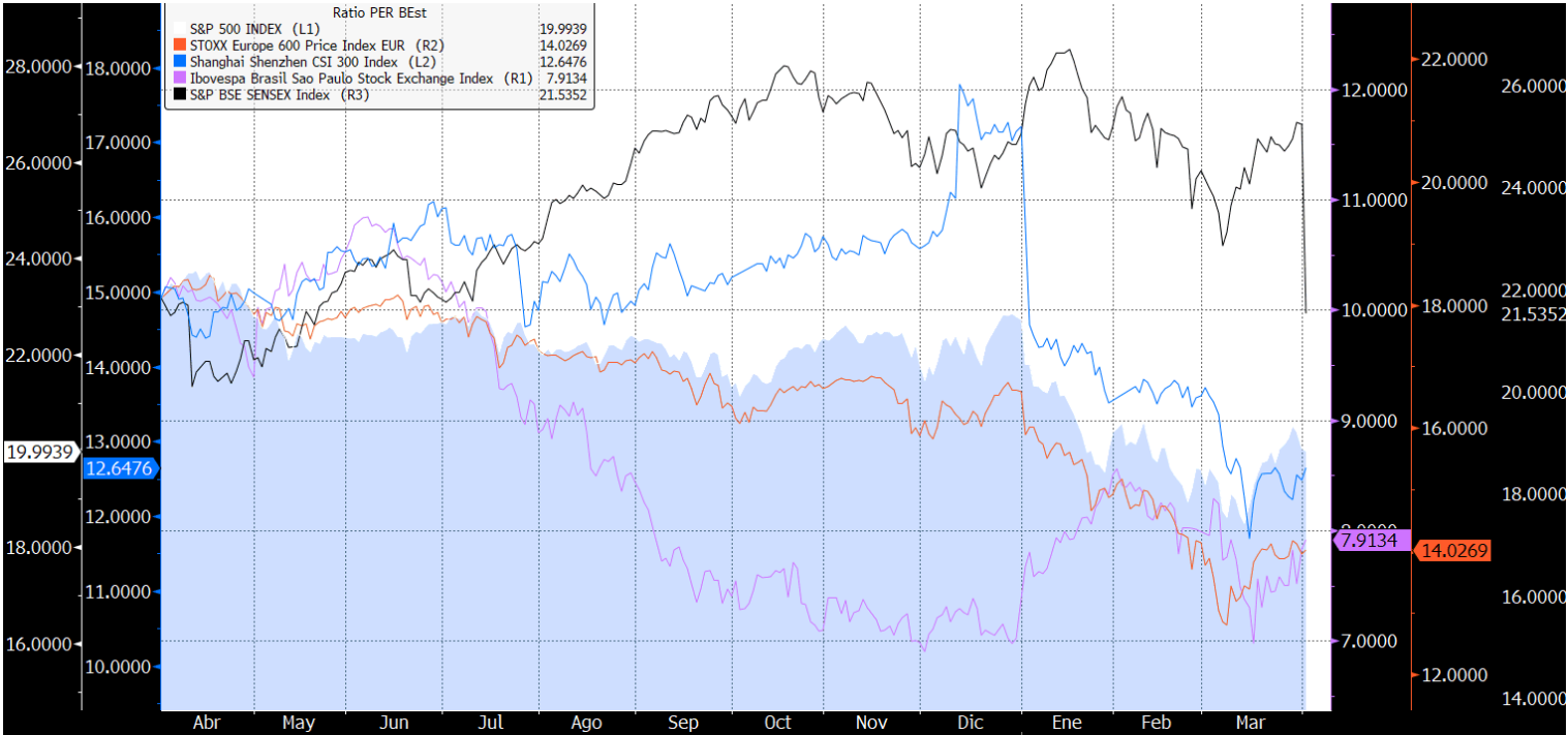
PER de países desarrollados y emergentes
